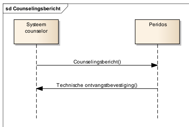
Figuur 4: Sequentiediagram van het counselingsbericht
