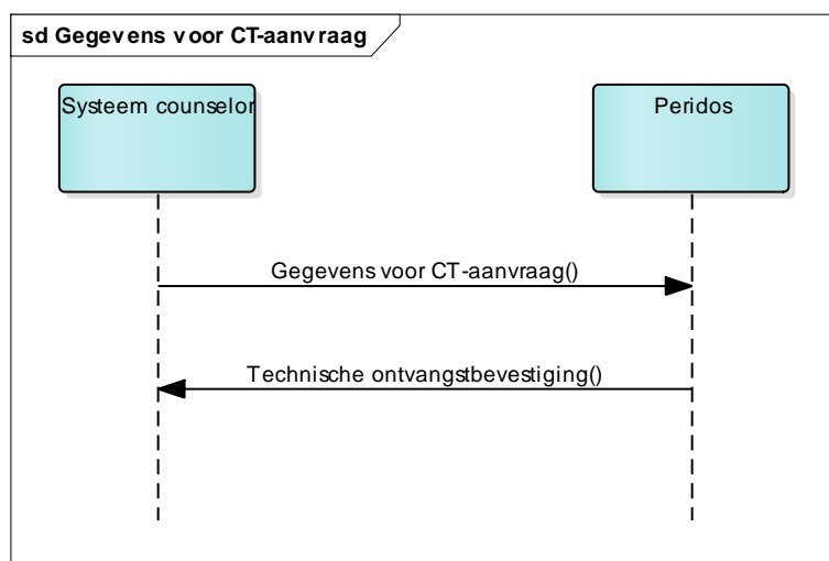
Figuur 4: Sequentiediagram van Gegevens voor CT-aanvraag
