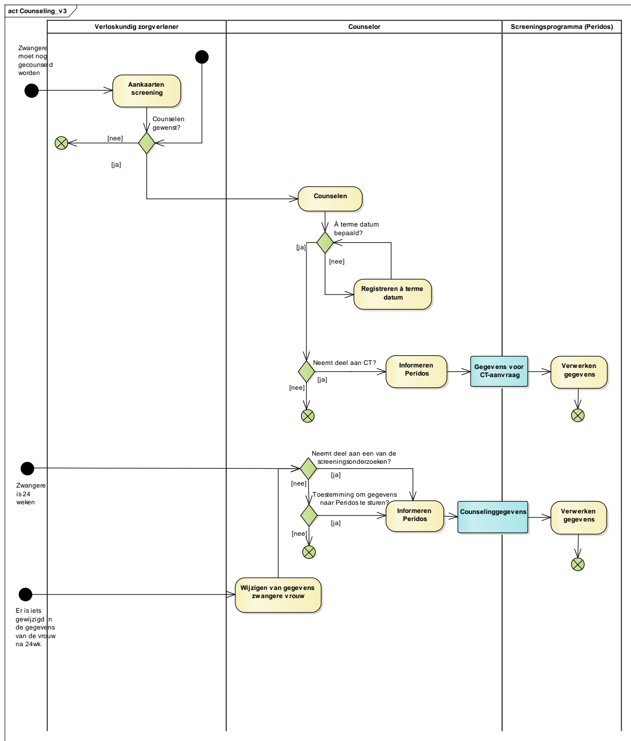
Figuur 2: Activiteitendiagram van het counselingsproces
