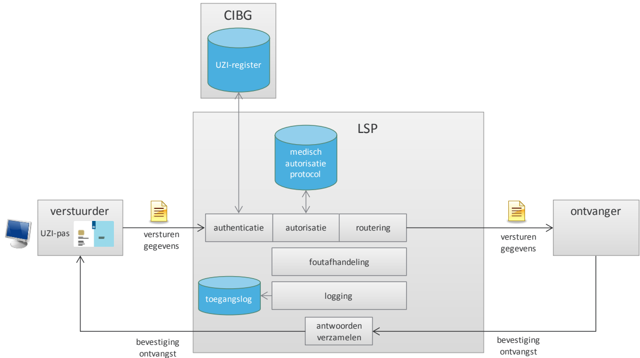
Figuur 21 - Het LSP voor PUSH verkeer (versturen)
