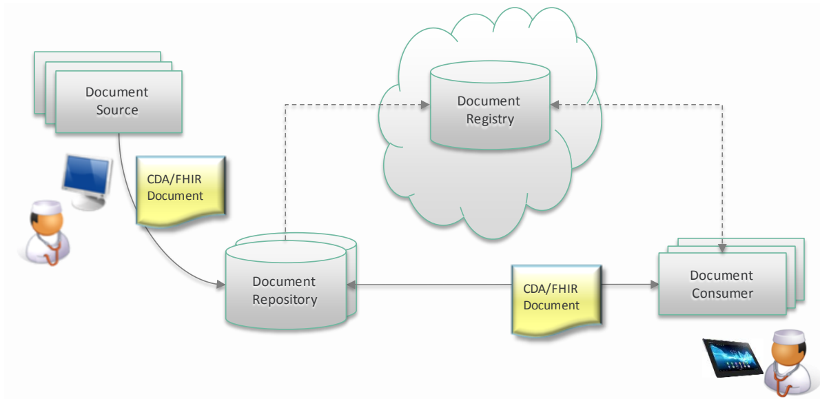
Figuur 17 - De werking van een XDS omgeving
