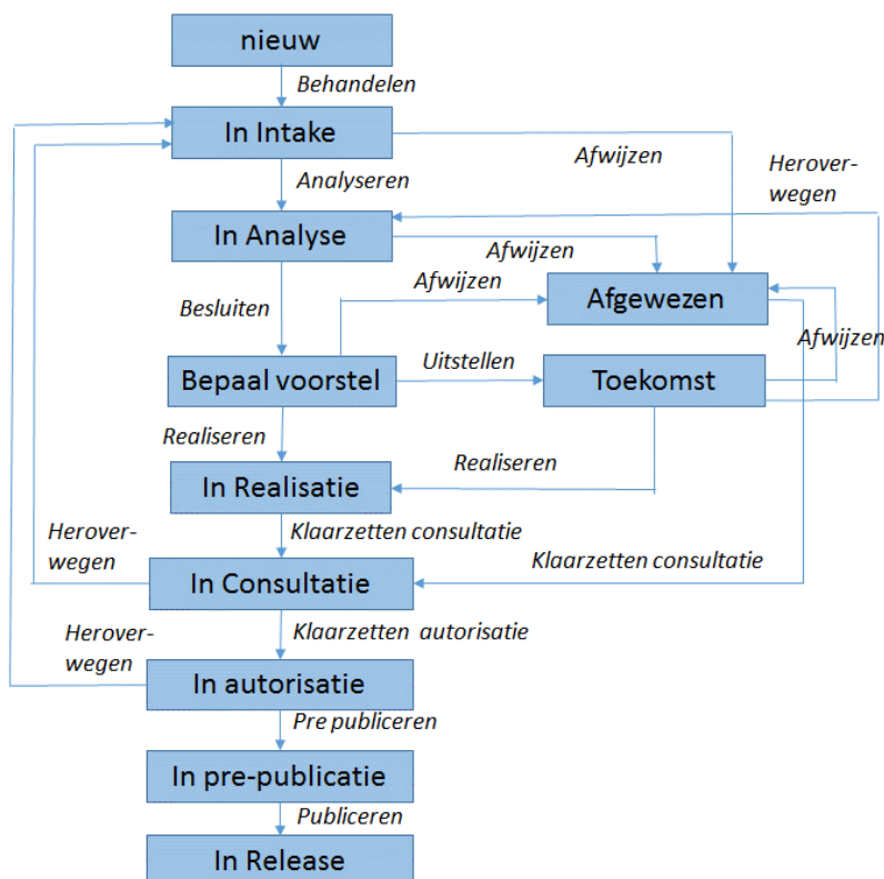
Figuur 3: Processtappen en statussen in beheerproces zibs
